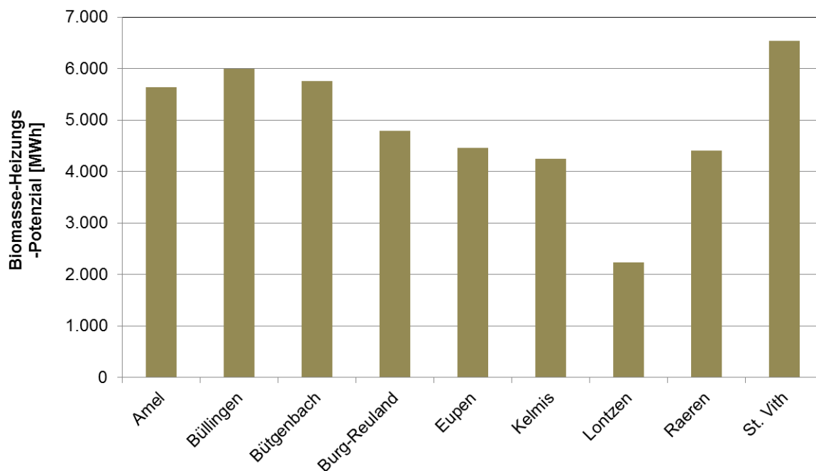
Abbildung 22: Potenziale Pelletkessel in der Deutschsprachigen Gemeinschaft, Beitrag zur Wärmeerzeugung
