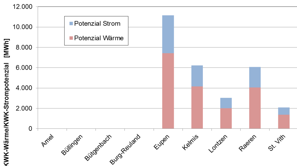
Abbildung 24: KWK-Potenziale in der Deutschsprachigen Gemeinschaft, öffentliche Gebäude (oben) und Sonstige (unten) pro Jahr
