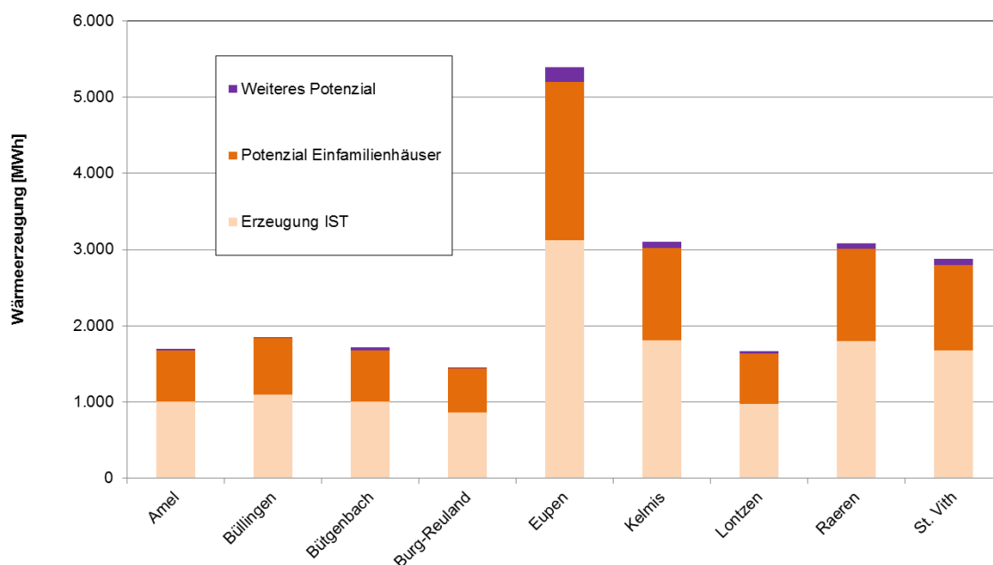
Abbildung 21 : Solarthermie-Potenziale in der Deutschsprachigen Gemeinschaft
