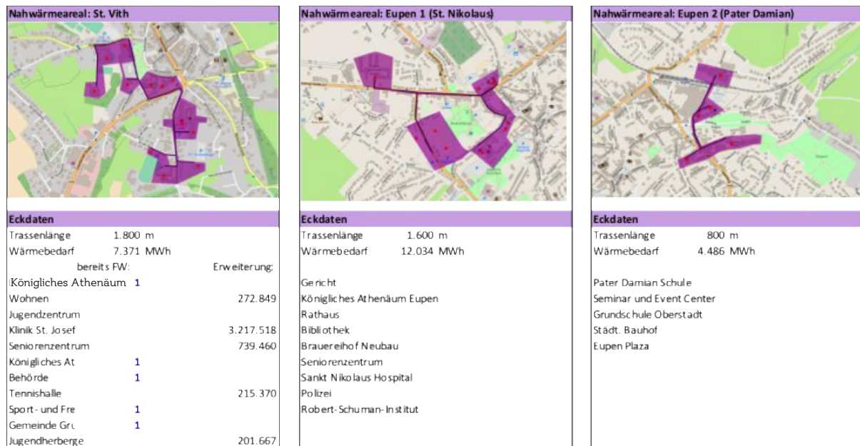
Abbildung 25 : Nahwärmepotenziale in der Deutschsprachigen Gemeinschaft
