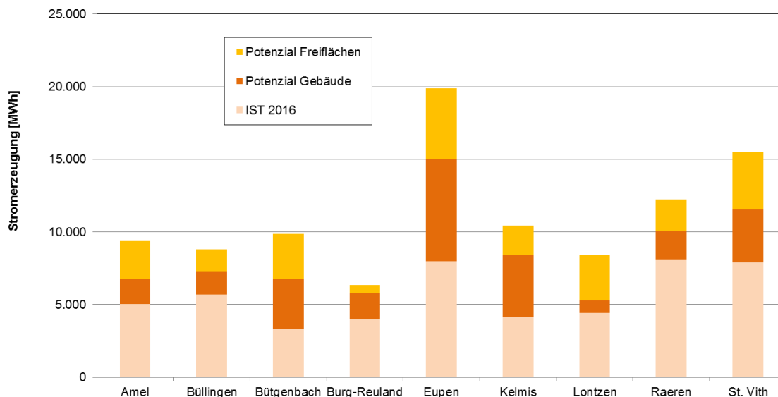
Abbildung 20 : PV-Potenziale (Stromerzeugung pro Jahr) in der Deutschsprachigen Gemeinschaft, IST, Ausbau Gebäude und Freiflächenpotenzial.
