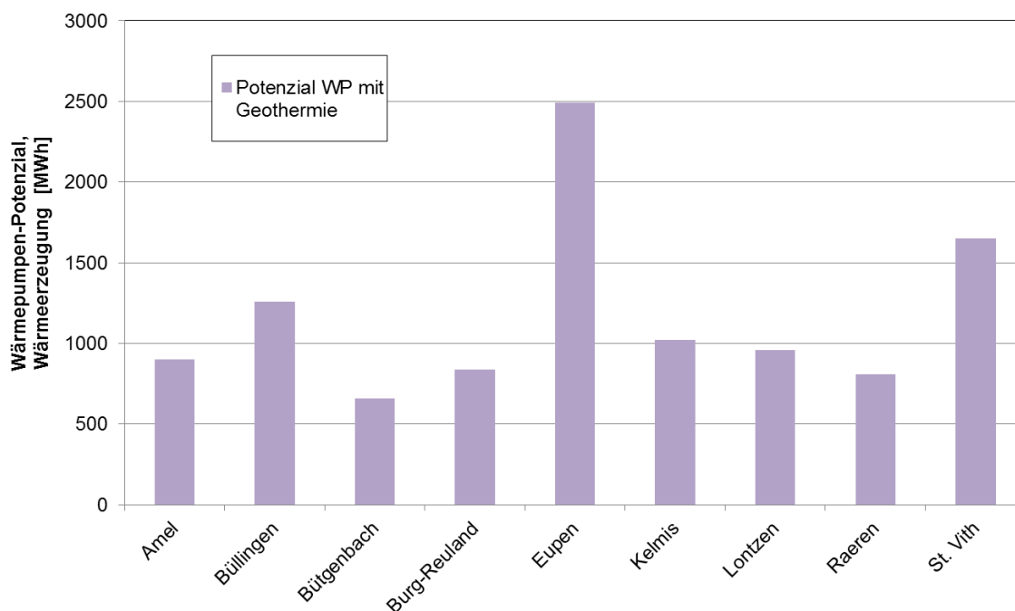
Abbildung 23: Potenziale geothermische Wärmepumpen, Beitrag zur Wärmeerzeugung
